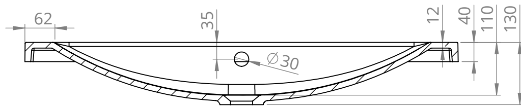
PRZEKRÓJ N-N SKALA 1 : 8
